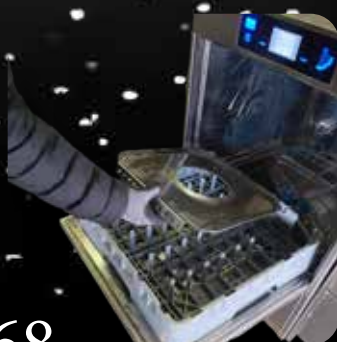
Bandeja extraíble y embutida de una sola pieza, sin soldaduras. Construida en acero inox AISi-304, apta para el lavavajillas
